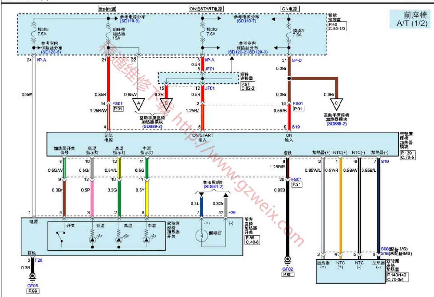
座椅加热器(1)
